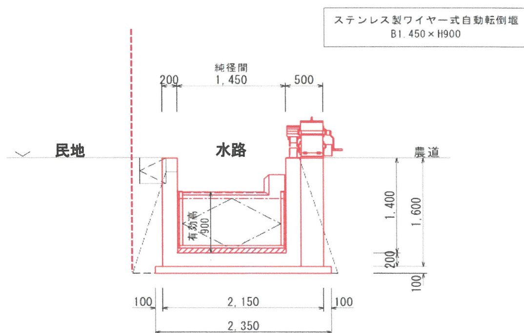
標準断面図
