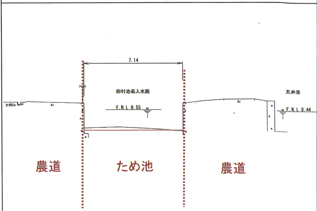
標準断面図
