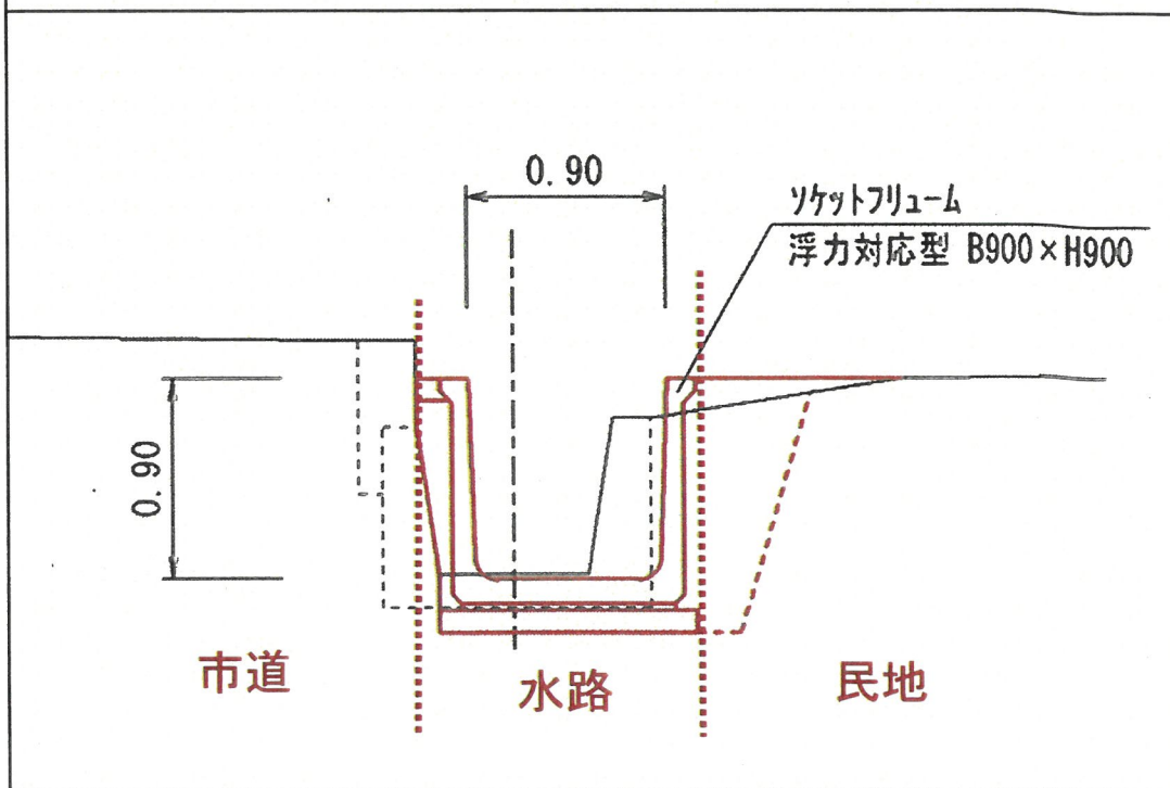
標準断面図
