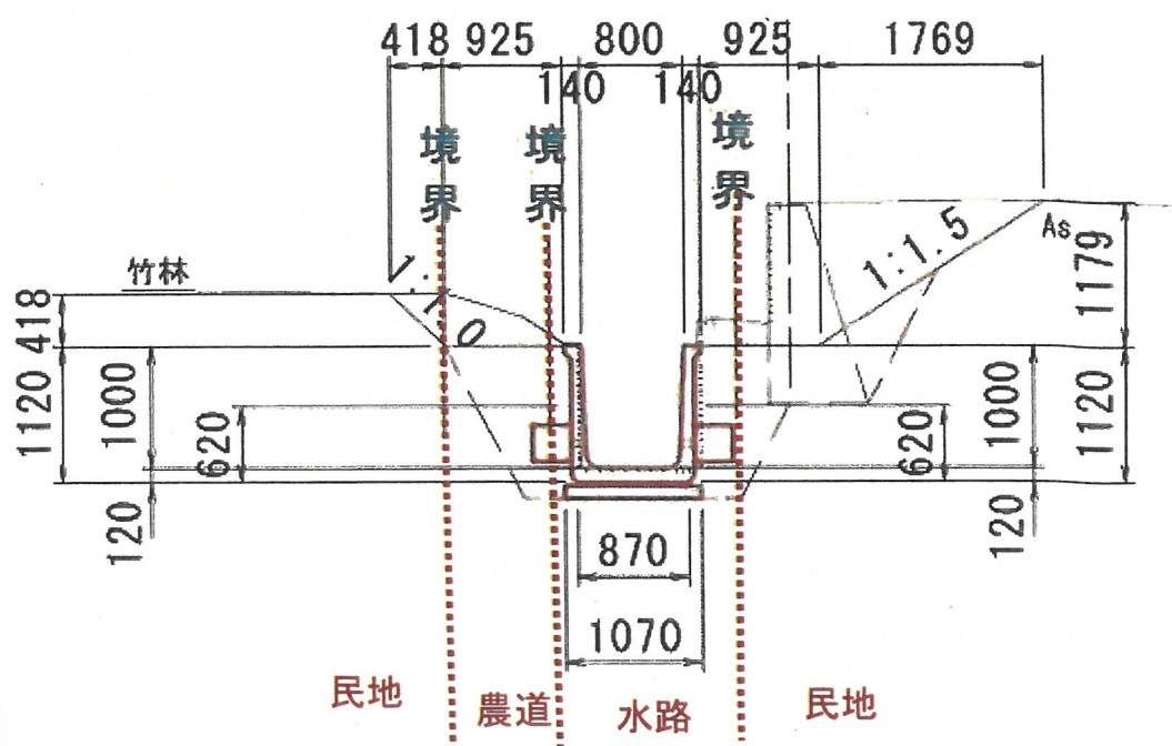
標準断面図
