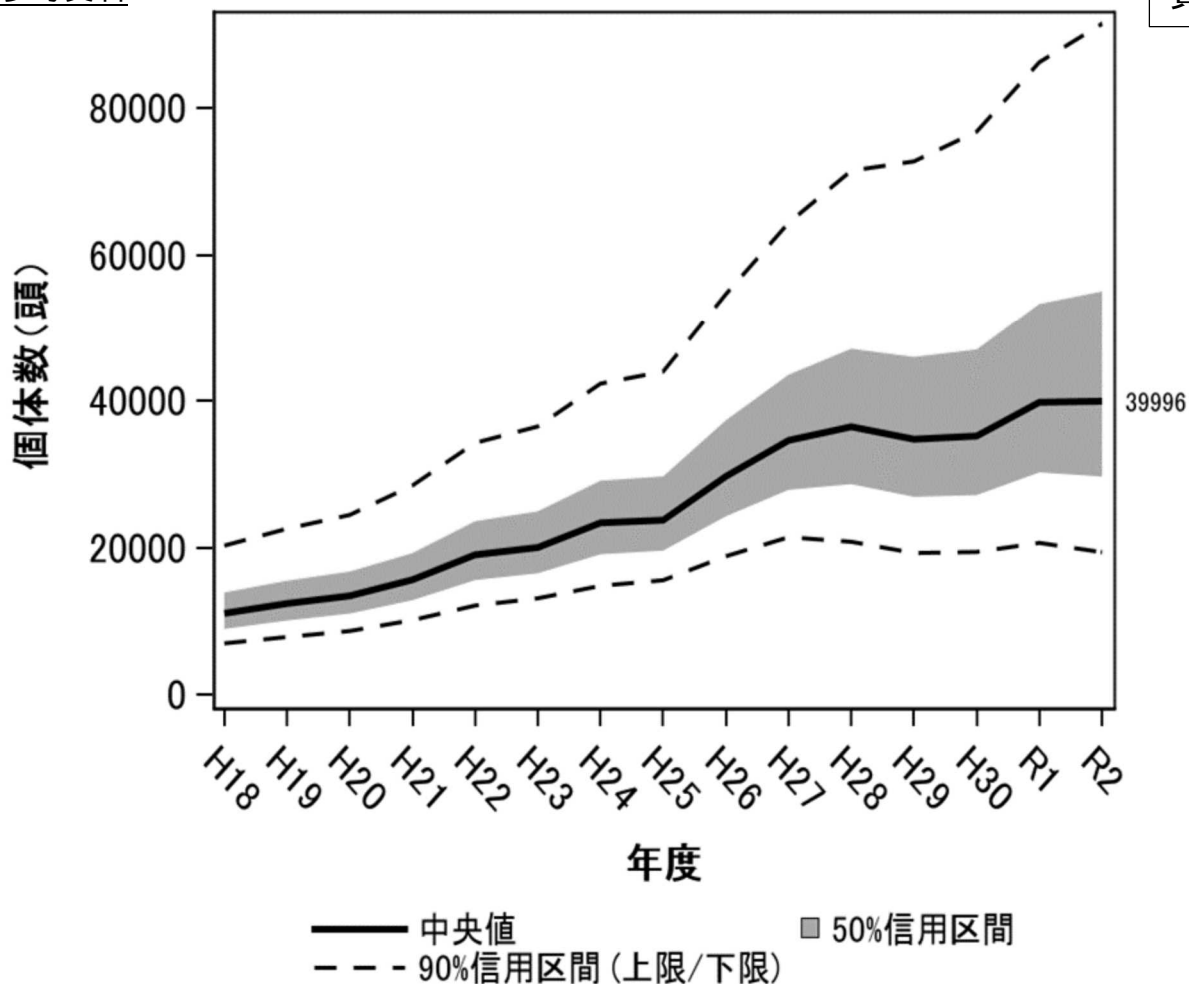
図 1 推定生息頭数の推移(本土部イノシシ)
