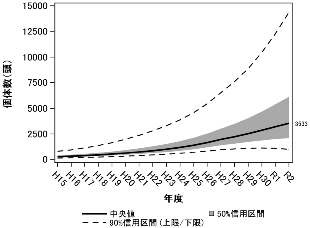
図3 推定生息頭数の推移(本土部ニホンジカ)
