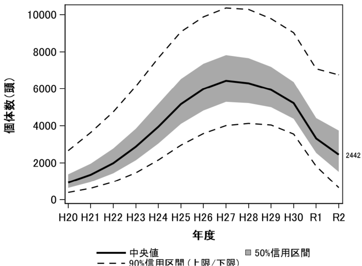
図 2 推定生息頭数の推移(小豆島イノシシ)
