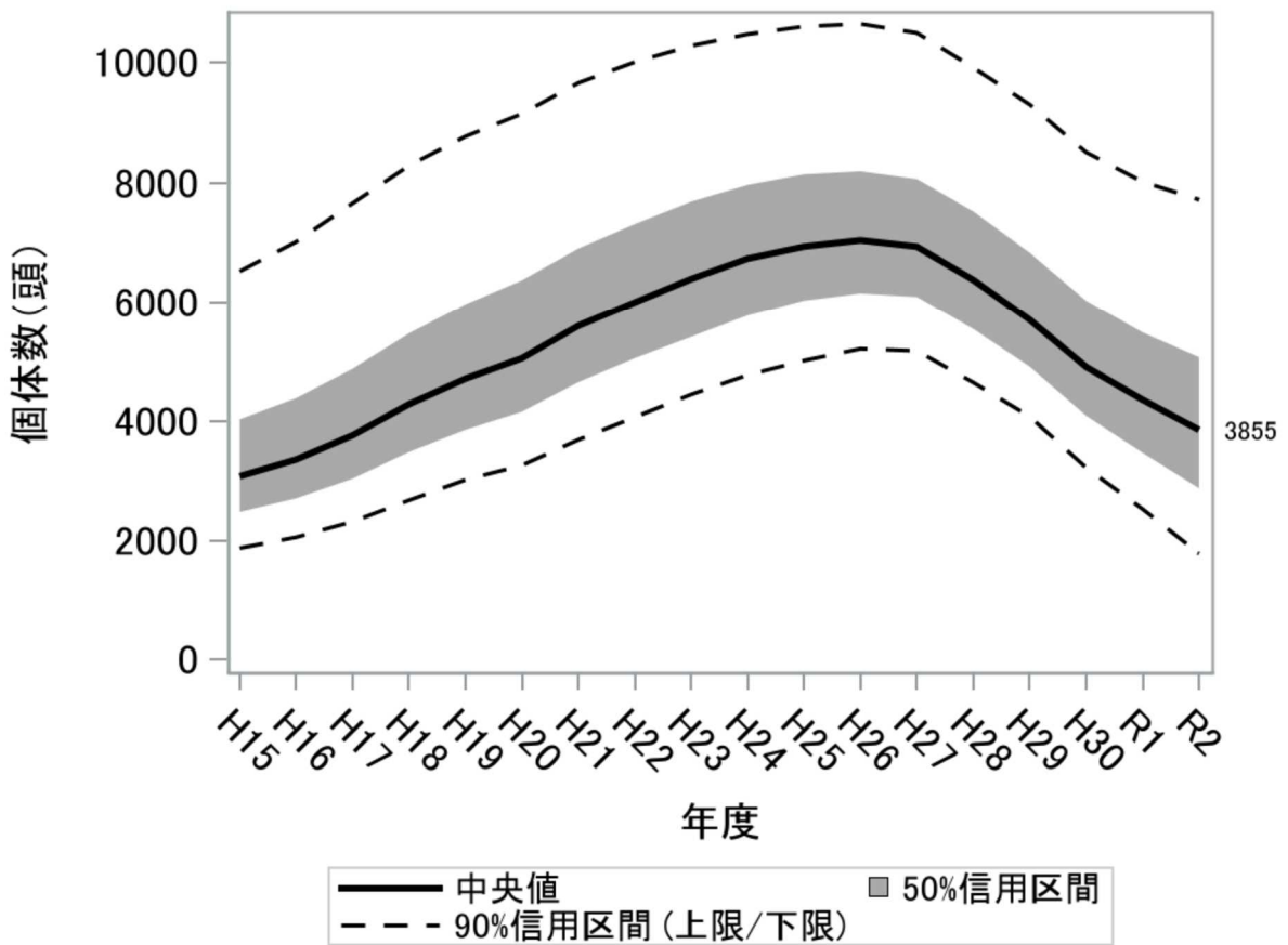
図4 推定生息頭数の推移(小豆島ニホンジカ)
