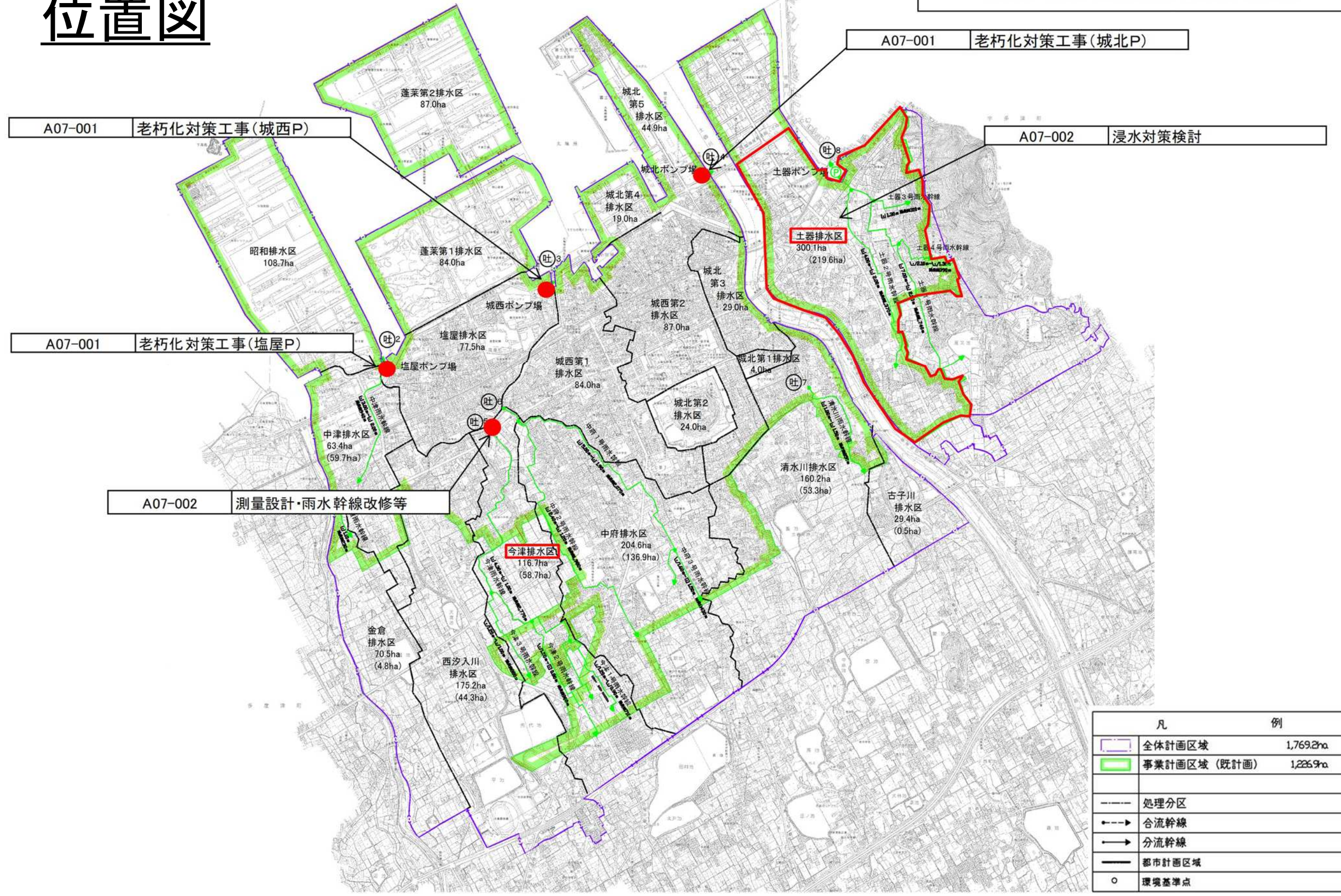
丸亀市下水道計画図(単独公共下水道)
