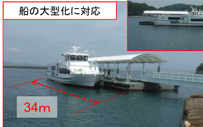
第2浮棧橋(整備後)
