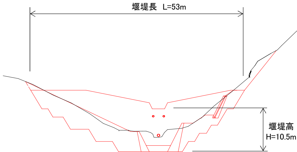
(堰堤正面図)
