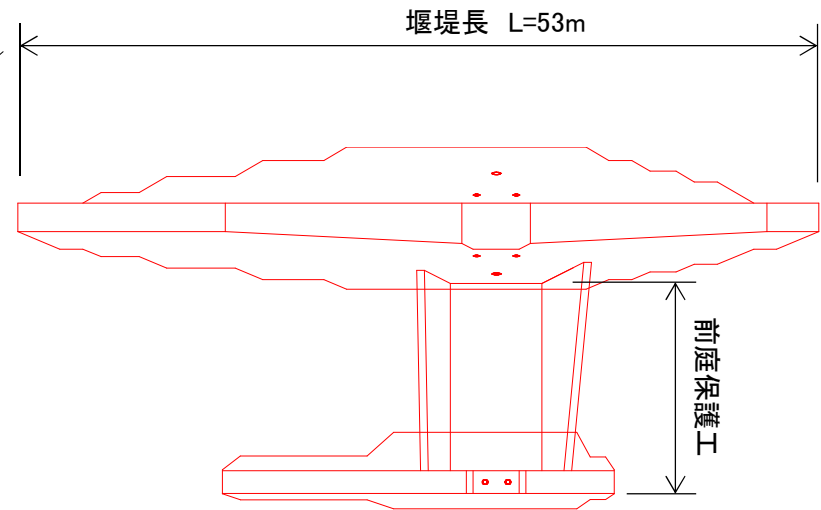
(堰堤平面図)
