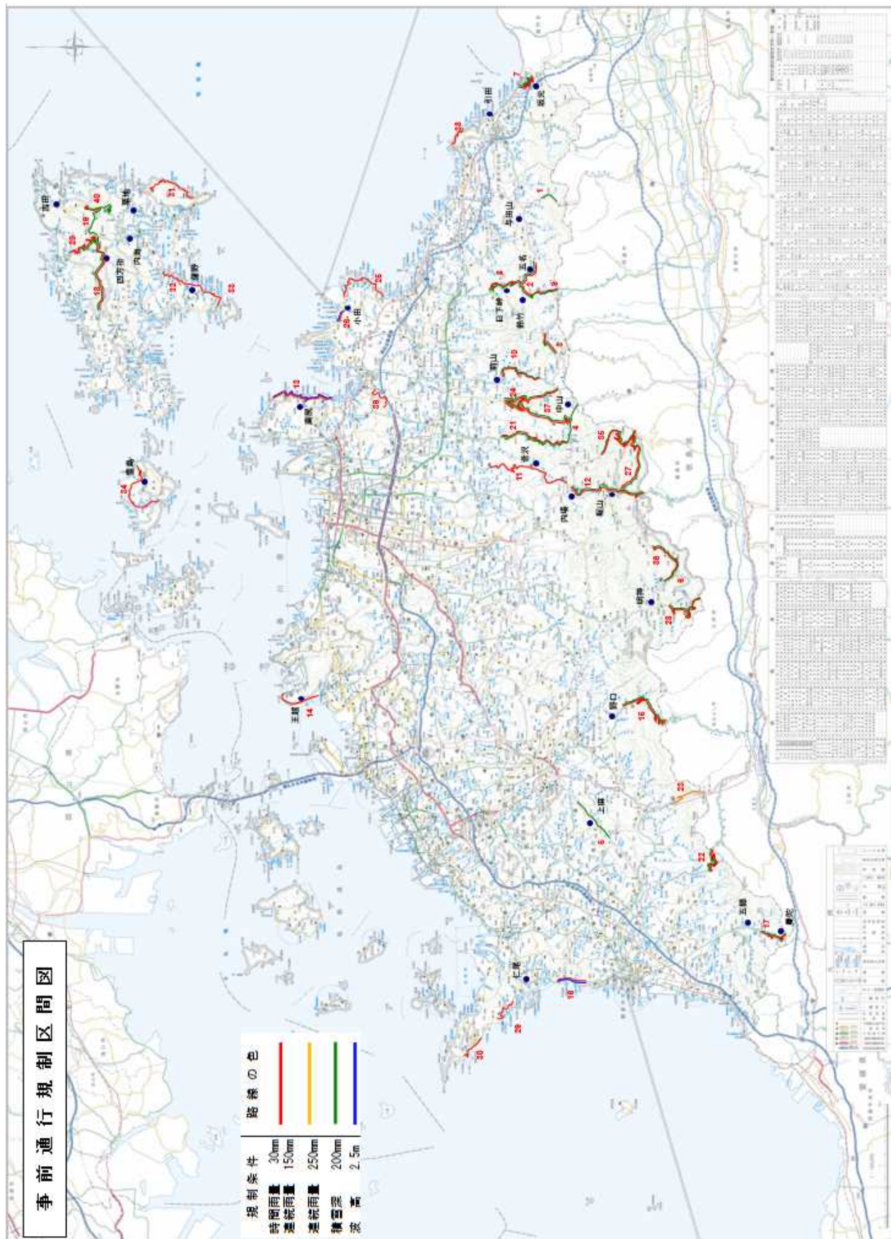
13-5 異常気象時道路通行規制箇所図
