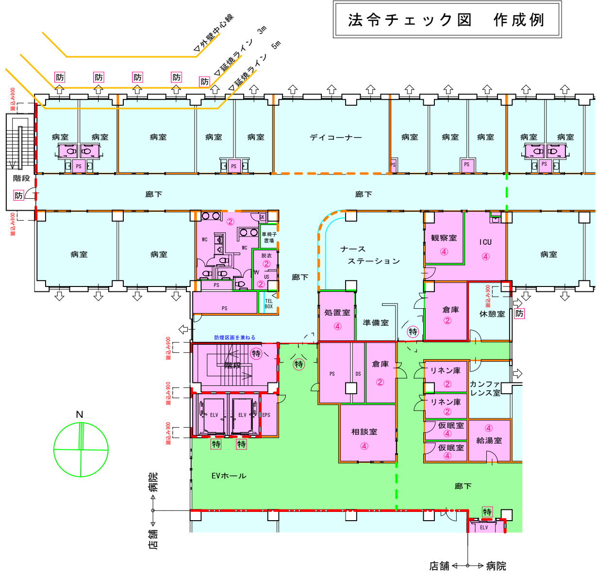
平面図 (S=1:200)
