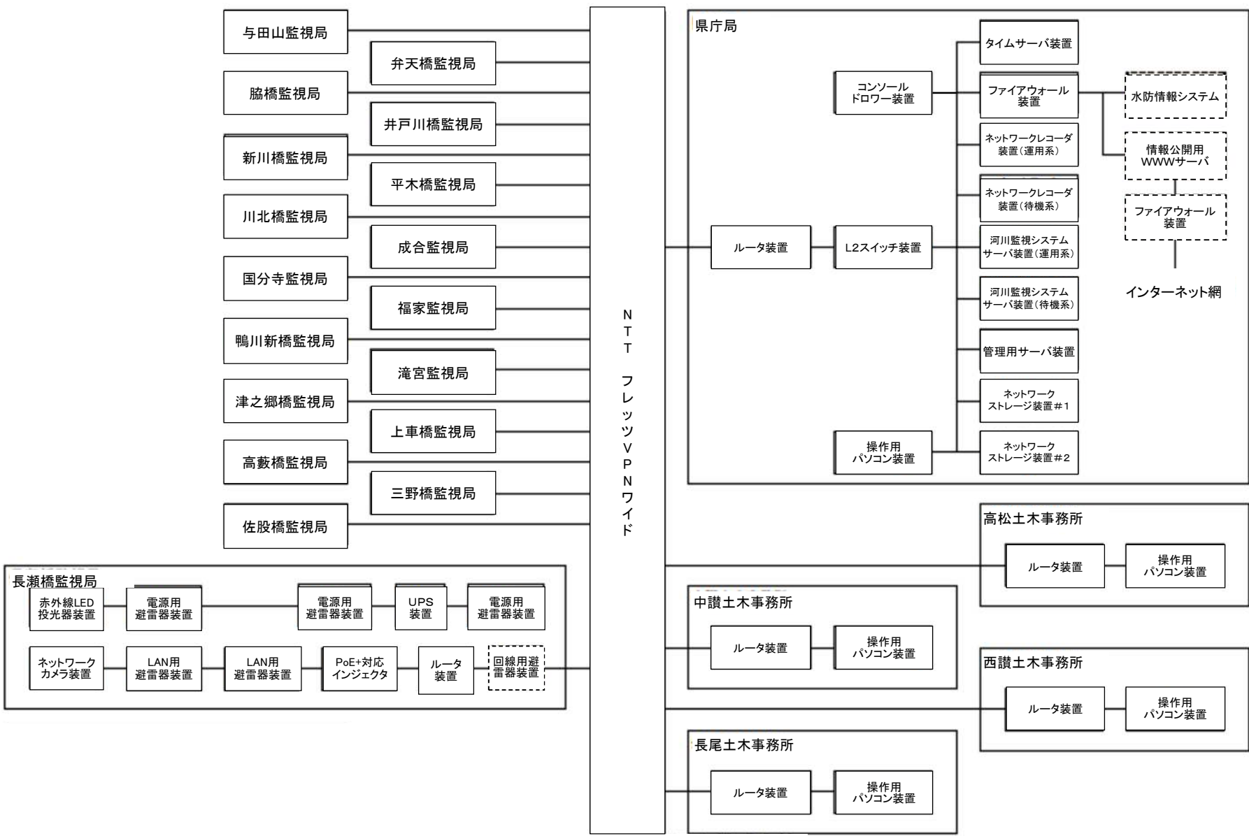
図 ー8 [ 河川監視システム構成図 ]
