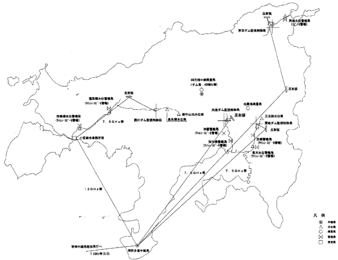
(2) 小豆総合管内多重無線系統図
