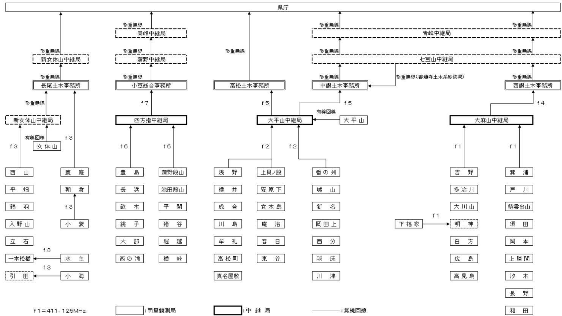
図-10 香川県砂防情報システム系統図
