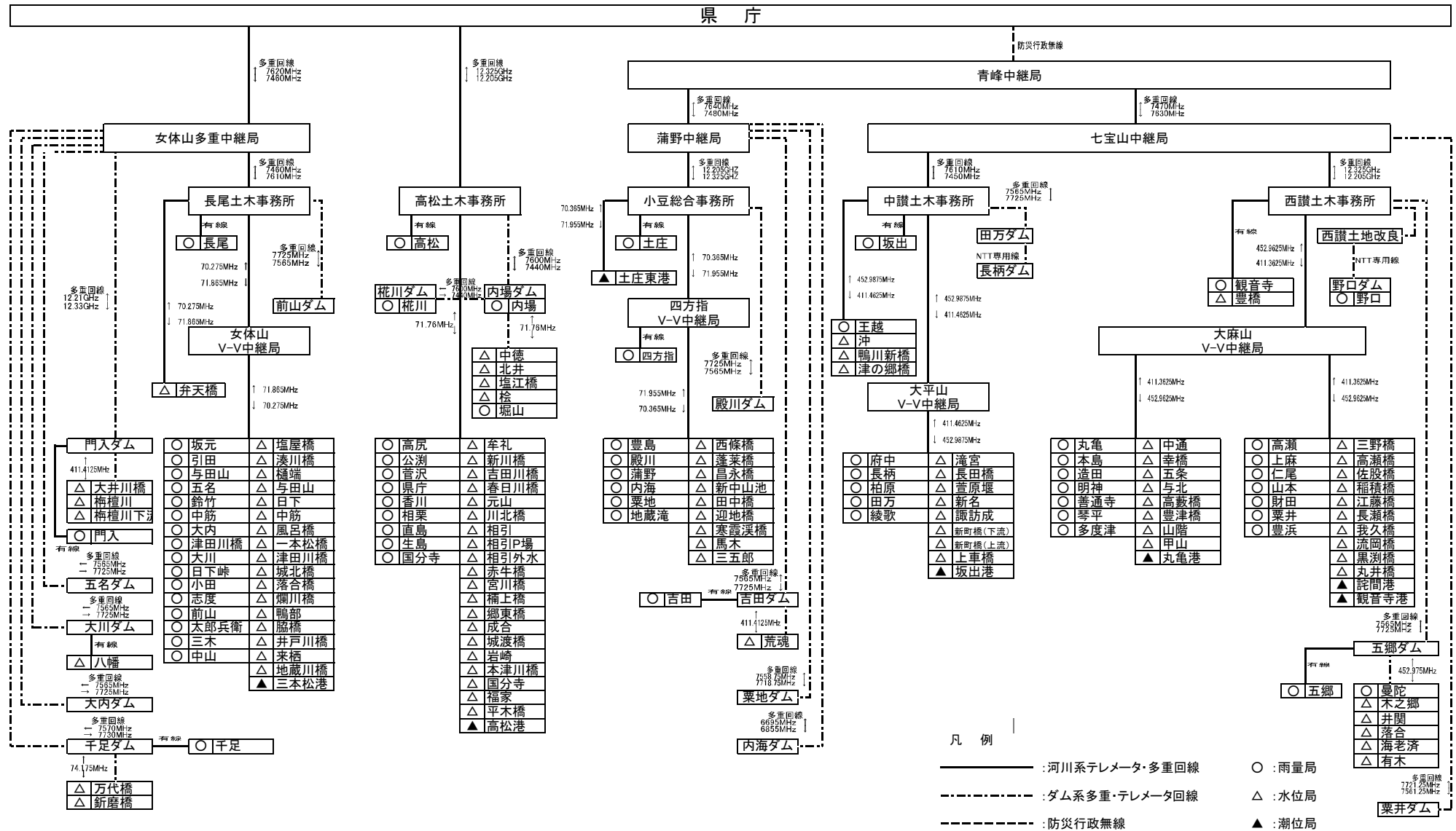
図 一7 [ テレメータ回線構成図 ]
