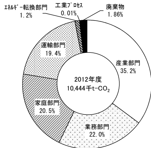
図2-5 CO 2 排出量の内訳（部門別）
