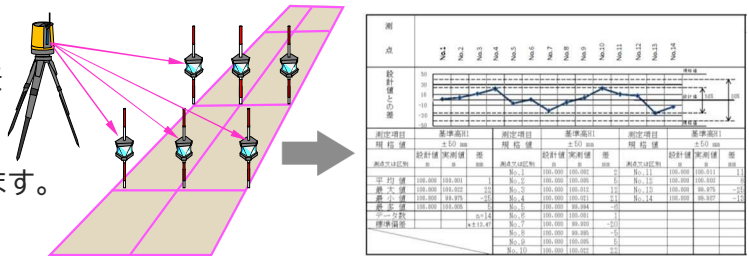
舗装工 3次元出来形管理等の施工管理で適用できる3次元計測技術
