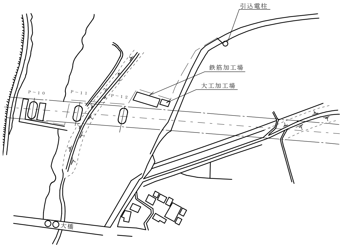
図二 仮設電気設備配置図
