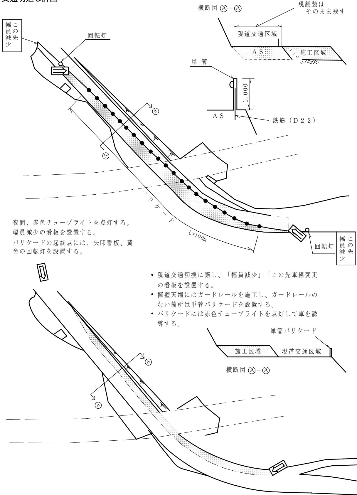
図-5 現道交通切替及び夜間の安全施設計画 (〇〇/〇〇~〇〇/〇〇)
