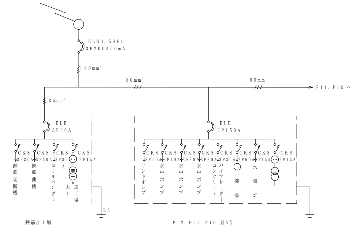
図一 仮設電気設備単線結線図
