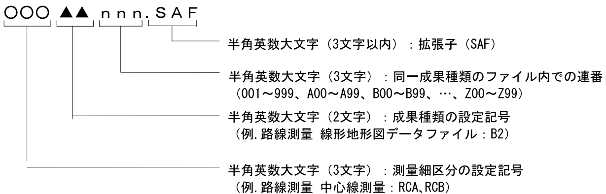
図 2 SAF ファイルの命名規則
