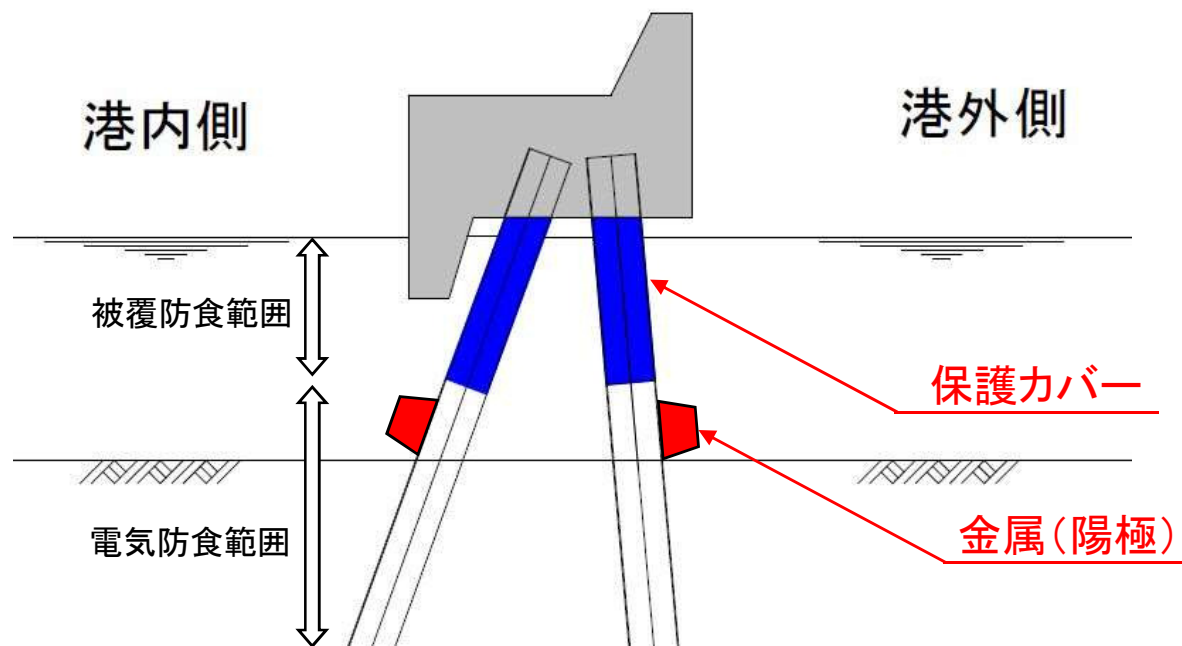
横断面図
