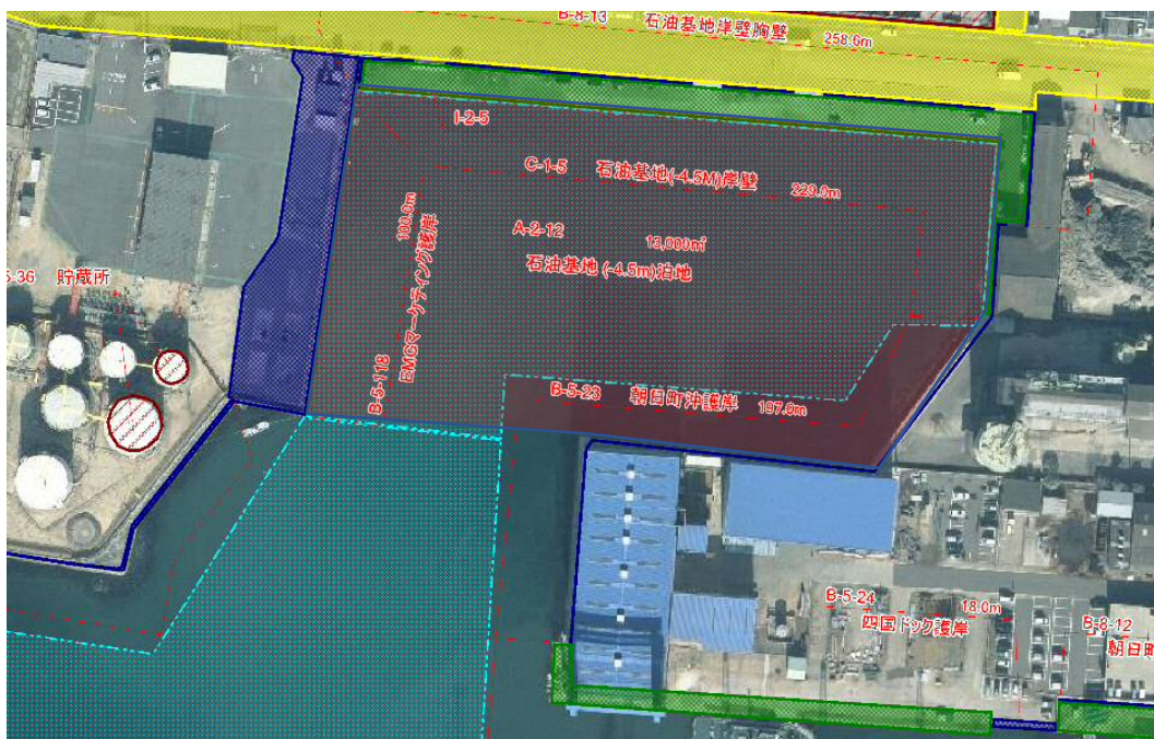
図 II-1-4 石油基地(-4.5m)岸壁及び隣接護岸等の整備位置
