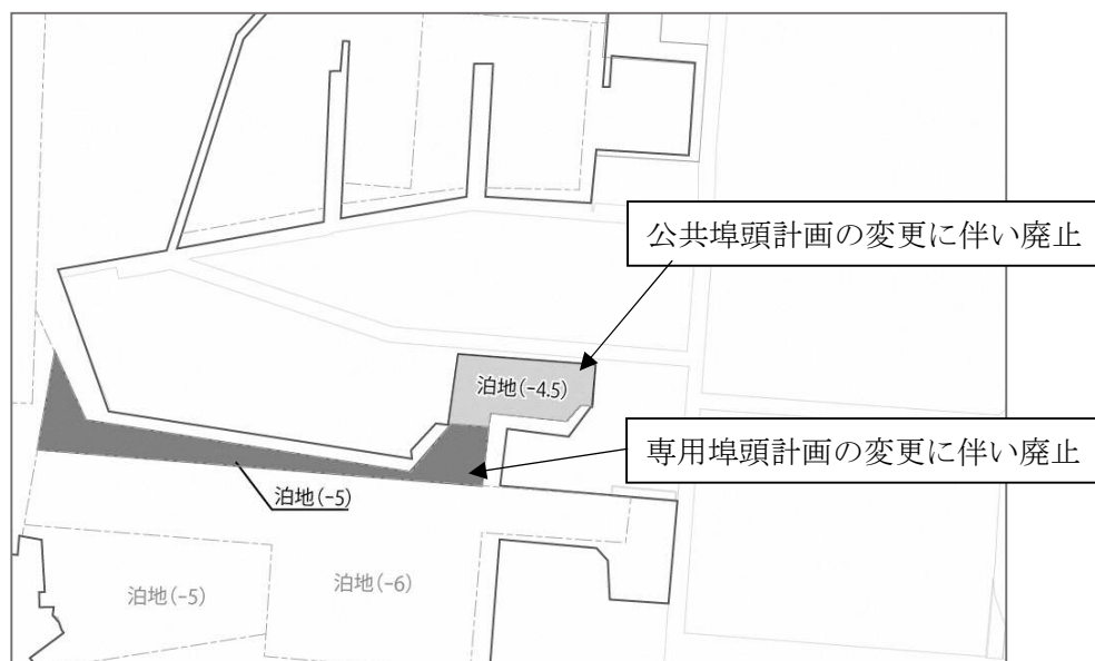
図Ⅱ-3-1 廃止する水域施設の位置
