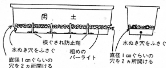
図-2 底面吸水プランター
