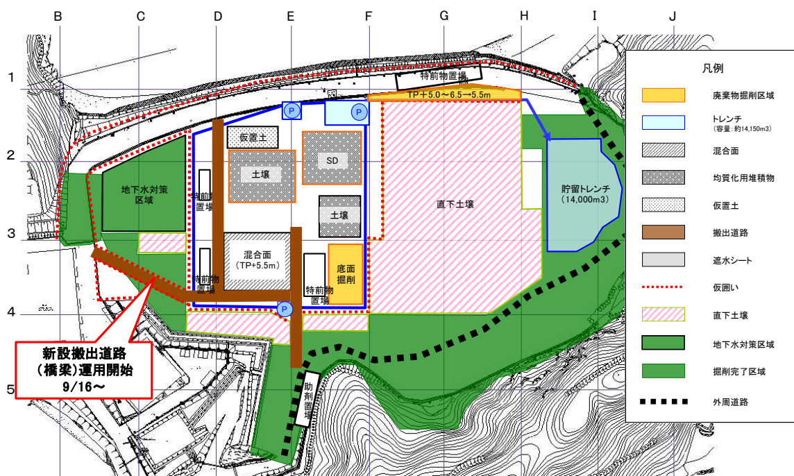
図1 平成27年9月掘削実績
