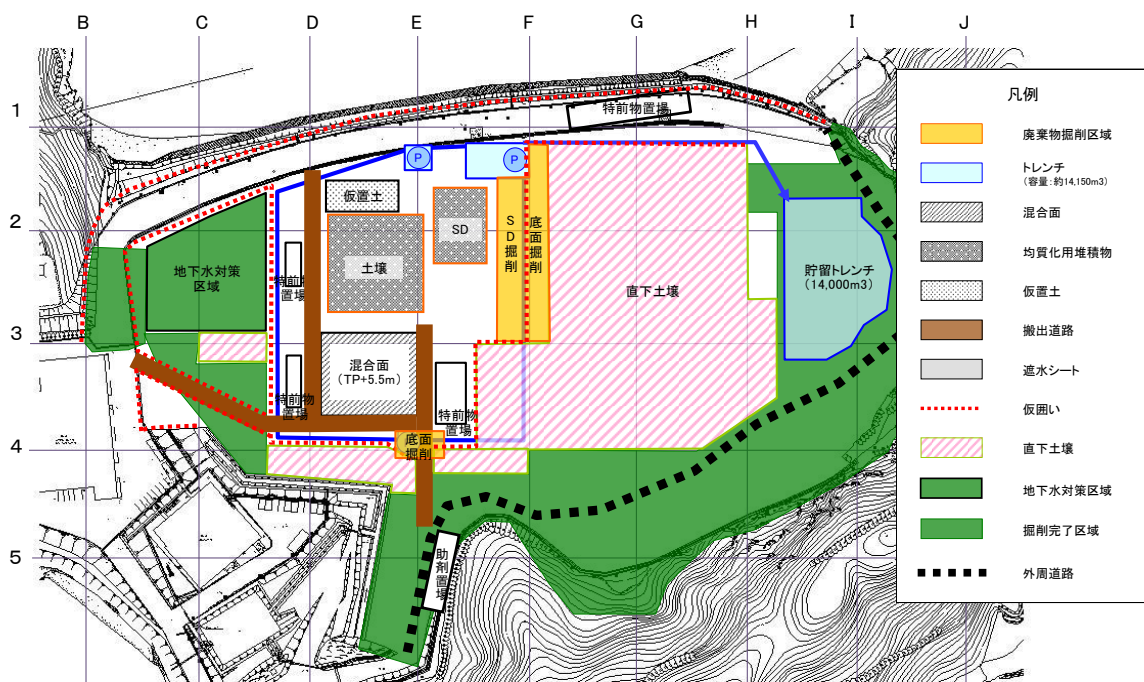
図2 平成27年10月掘削計画
