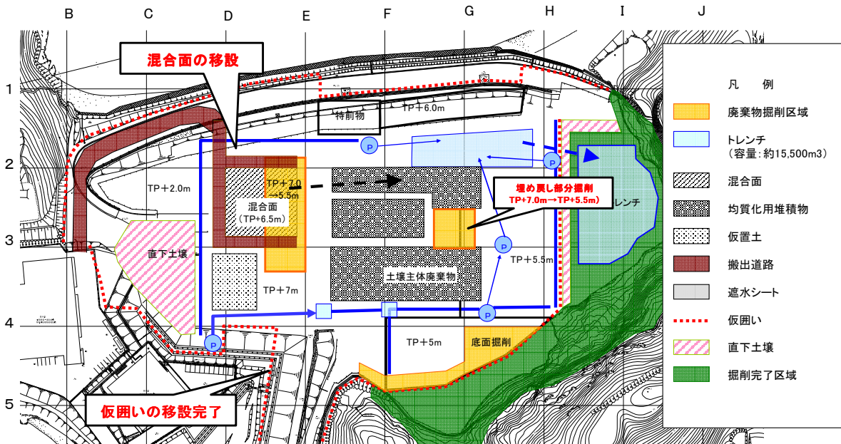
図2 平成26年1月掘削計画
