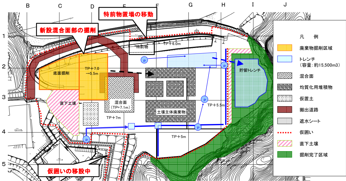
図1 平成25年12月掘削実績
