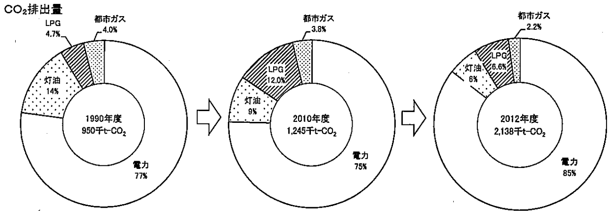
図 3-2-3-6 家庭部門のCO 2 排出量の電力由来構成比
