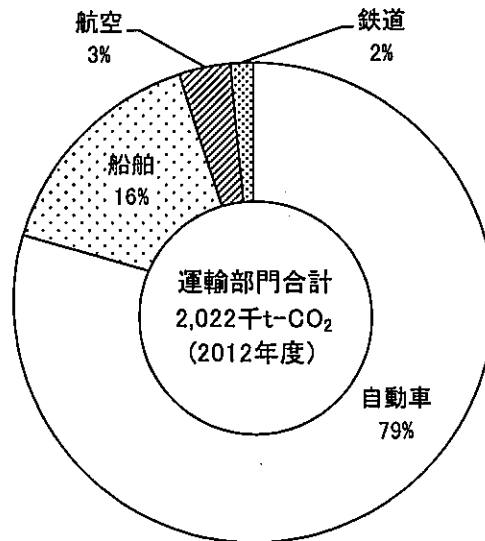
図 3-2-4-2 運輸部門のCO 2 排出量の構成割合（輸送機関別）
