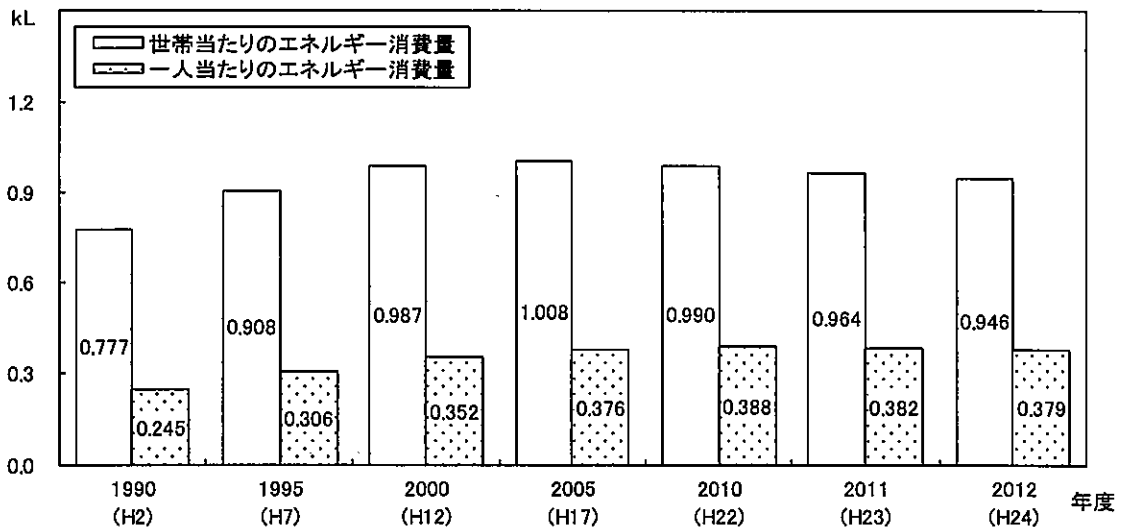
図 3-2-3-5 世帯及び人口当たりのエネルギー消費量の推移
