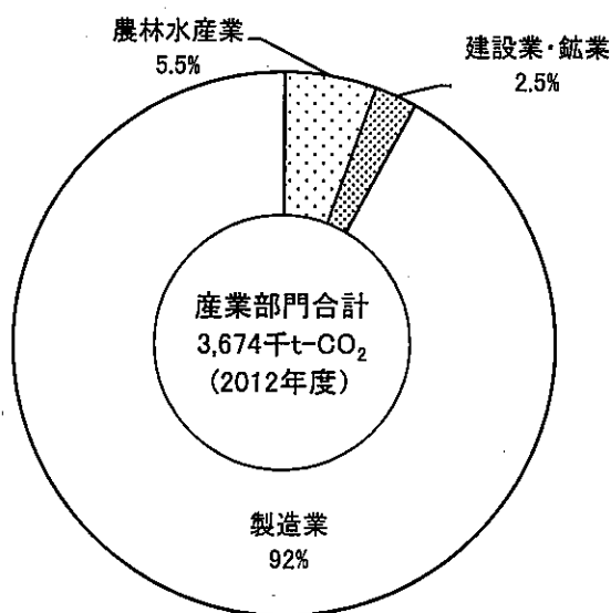
図 3-2-1-1 産業部門のCO 2 排出量の構成割合(業種別)
