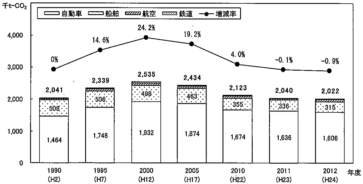
図 3-2-4-1 運輸部門のCO 2 排出量の推移
