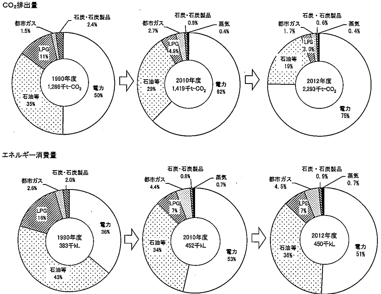
図 3-2-2-3 業務部門のCO 2 排出量及びエネルギー消費量の構成割合(燃料種別)
