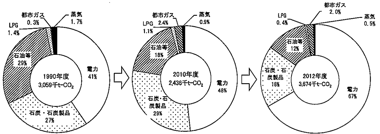
図 3-2-1-2 産業部門のCO 2 排出量及びエネルギー消費量の構成割合(燃料種別)
