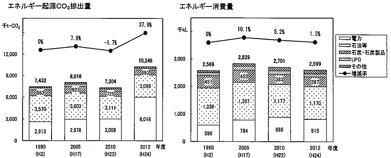
図 3-2-4 エネルギー起源CO 2 排出量とエネルギー消費量の推移(燃料種別)
