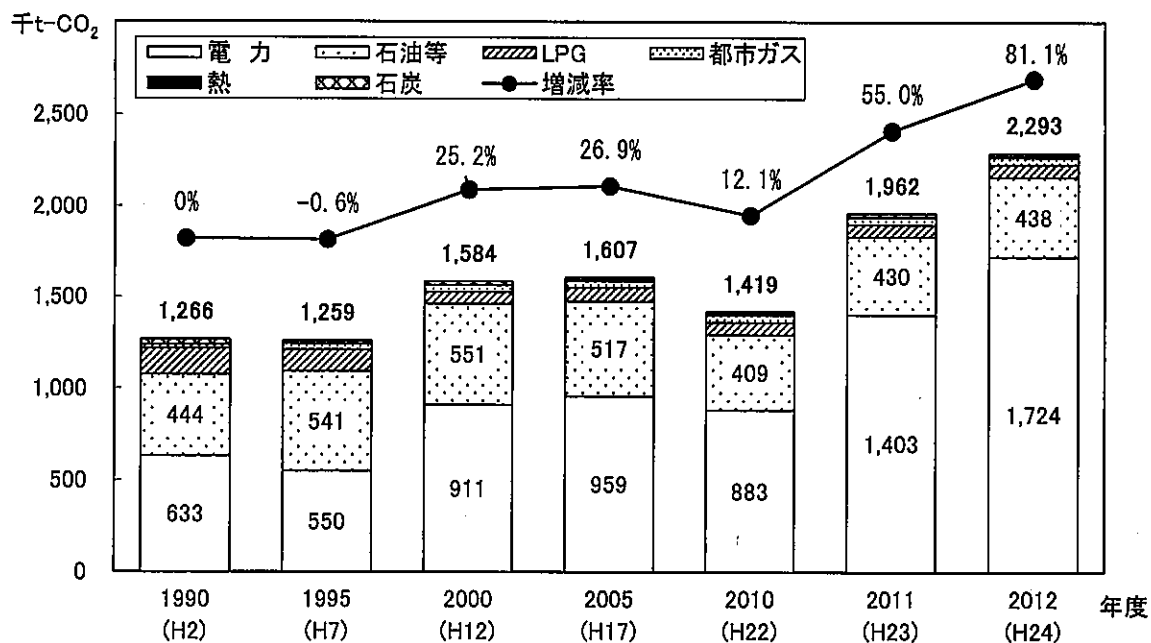
図 3-2-2-1 業務部門のCO 2 排出量の推移
