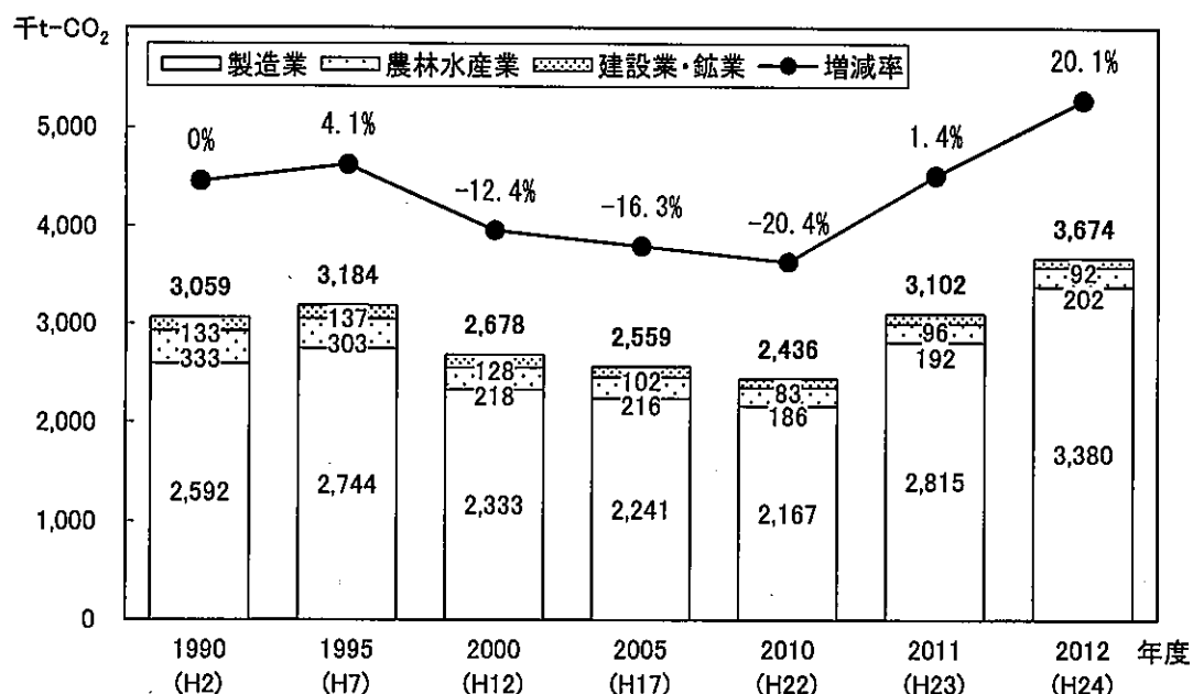
図 3-2-1-1 産業部門のCO 2 排出量の推移
