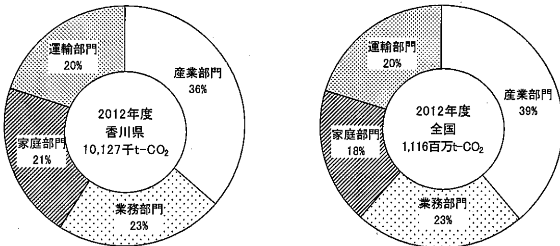
図 3-2-2 香川県と全国のCO 2 排出量の構成割合(部門別)
